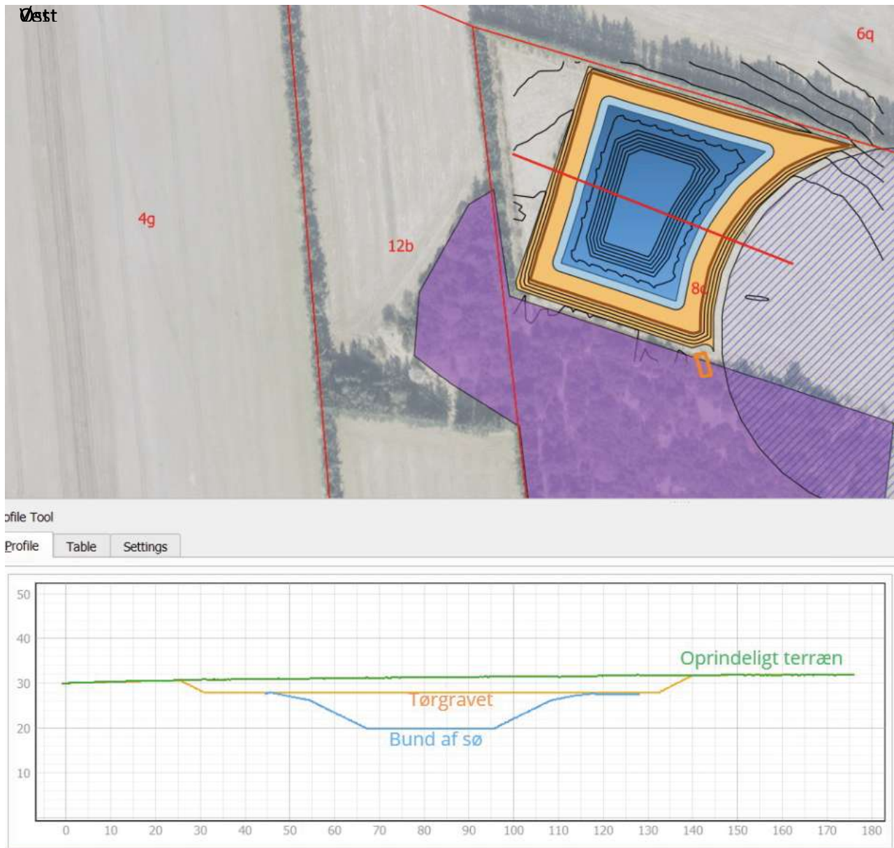
Figur 4: Profil gennem færdiggravet sø. Højdekurver 1 m. Søen er opbygget som vist på fig. 2. Profilet er uden overhøjning. Mørkeblå er sø med 15 m's afstand til skræntfod. Lyseblå med 10 meters afstand.
