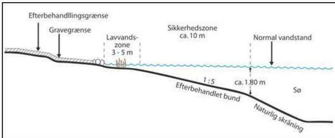
Figur 2: Principskitse for efterbehandling til sø
