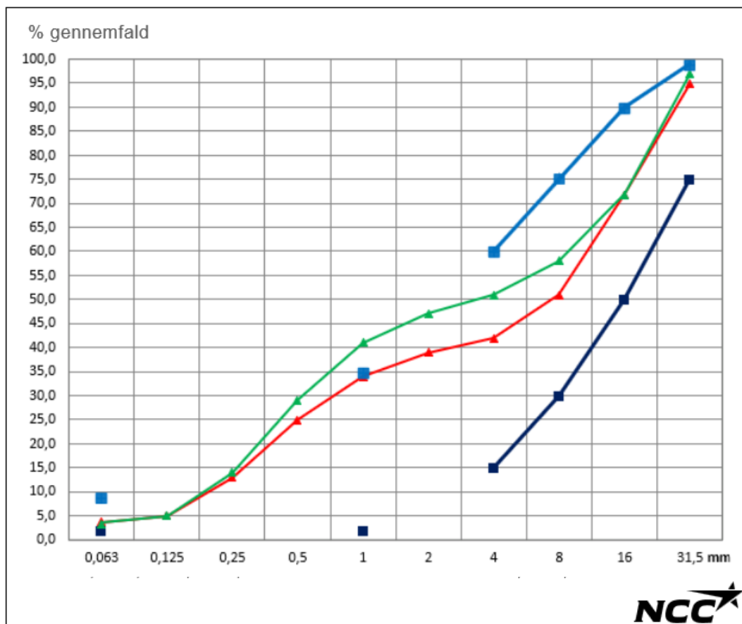
Figur 14. Kornstørrelsesfordelingen for SG II (rød) og Nyt Stabilt Grus (grøn) samt vejreglernes øvre krav for SG II (blå) og vejreglernes nedre krav for SG II (sort). Bemærk at grænsekurverne for øvre og nedre krav for SG II ikke er tegnet helt igennem. Det skyldes, at der i vejreglerne kun er fastsat krav i de fremhævede punkter. Der er valgt ikke at anvende fuldt optrukne grænsekurver, da det vurderes ikke at være korrekt iht. vejreglerne (ref. 2).
