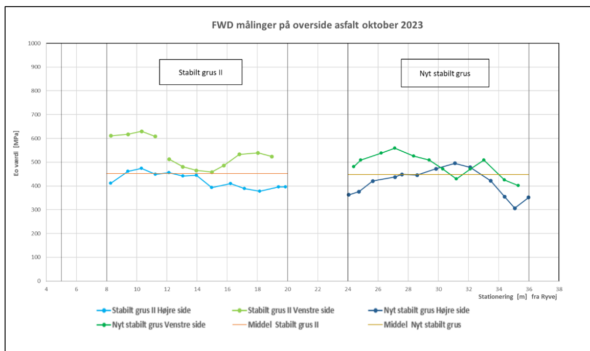
Figur 18. Overflade E-modulet, E_o , målt med stort faldlod (FWD) på oversiden af asfalten på prøvestrækningen i råstofgraven. Målt den 3. oktober 2023. Prøvefeltet "Stabilt grus II", st. 8 – 20 m med middelværdi 478 MPa og prøvefeltet "Nyt Stabilt Grus", st. 24 – 36 m med middelværdi 448 MPa. Området st. 0 – 5 m er overgangzone over grøft i indkørslen, området st. 5 – 8 m er overgangzone til prøvestrækningerne, området st. 20 – 24 m er overgangzone mellem prøvestrækningerne og området st. 36 – 40 m er overgangzone efter prøvestrækningerne.
