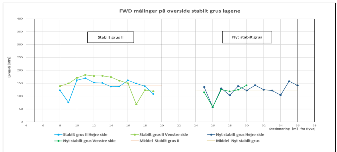
Figur 17. Overflade E-modulet, E_o , målt med stort faldlod (FWD) på stabilt grus overfladerne den 31. marts 2023. Prøvefeltet "Stabilt grus II", st. 8 – 20 m med middelværdi 143 MPa og prøvefeltet "Nyt stabilt grus", st. 24 – 36 m med middelværdi 120 MPa. Området st. 0 – 5 m er overgangzone over grøft i indkørslen, området st. 5 – 8 m er overgangzone til prøvestrækningerne, området st. 20 – 24 m er overgangzone mellem prøvestrækningerne og området st. 36 – 40 m er overgangzone efter prøvestrækningerne.
