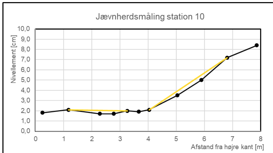
Figur 26 Sporkøring målt på SG II-feltet i forsøgsstrækningens station 10 m. Punkterne er opmålt med teodolit. Sporkøringen er den maksimale afstand mellem de opmålte punkter og det indlagte rethold (orange linje).
