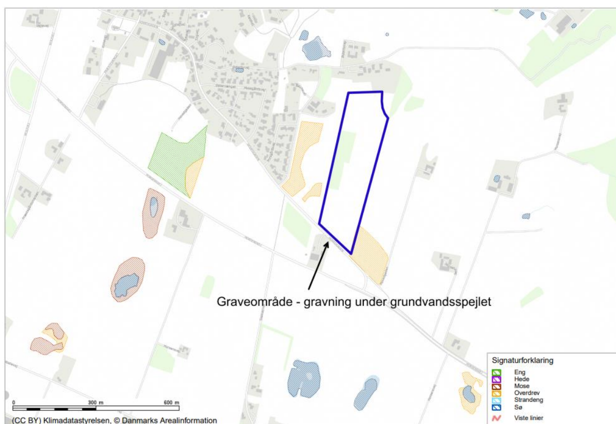
Figur 4 Kort over §3 beskyttede naturarealer i nærheden af graveområdet.
