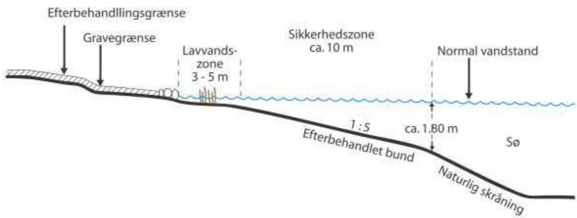
Figur 1 skitse af sø
