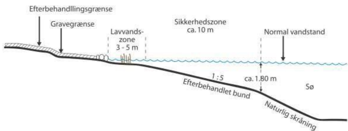
Figur.2 Principkitse for efterbehandling af søer.
